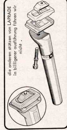
03321-LAPR = 47.45 orig. LAPRADE 606 EXTRA LEICHT UND ÜBERLANG = 200mm
