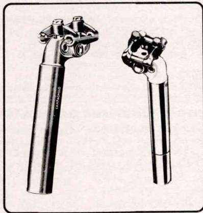
03332-CAZE = 41.- DM CAMPAGNOLO oder ZEUS -je nach lagerbestand- 25,8 bis 27,2 mit je 0,2 Ø
