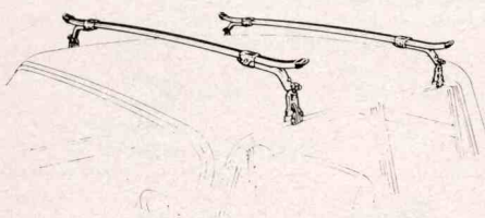
TRÄGERBRÜCKE in einfacher Ausführung zum Transport eines Tourenrades bzw maximal 2 Rennräder - Ausführung ähnlich obiger Abbildung
