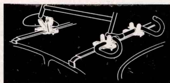
Modell "BLACK" Befestigung des Rades mit Riemen Garnitur für 1 Rad
